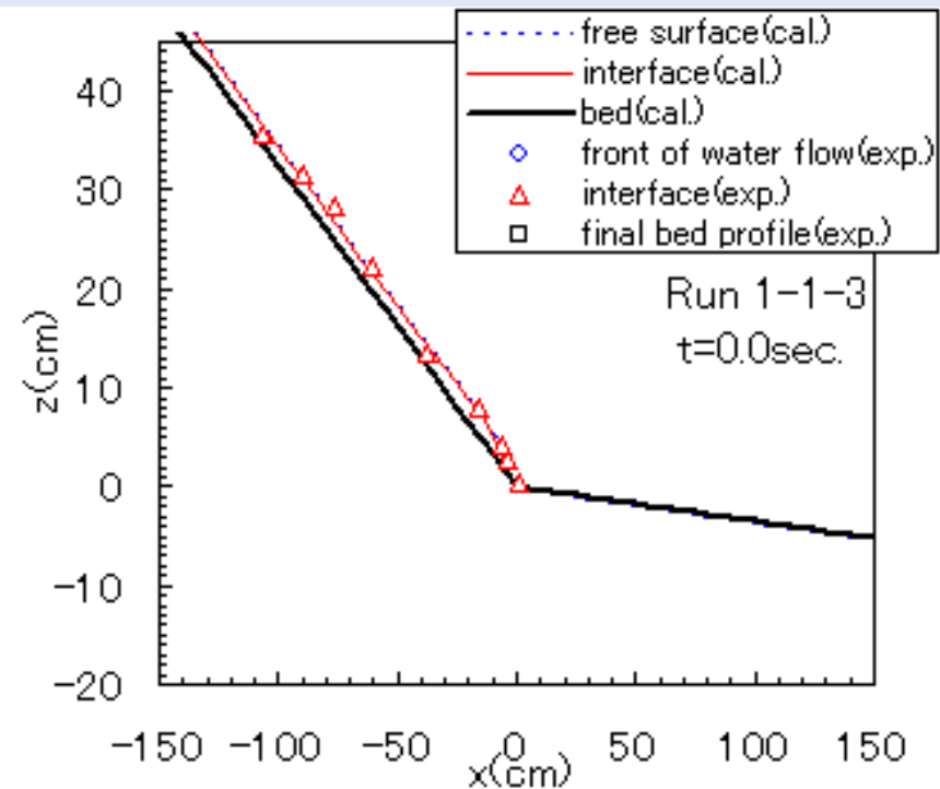
土石流の堆積過程に関する実験結果と数値計算結果との比較
