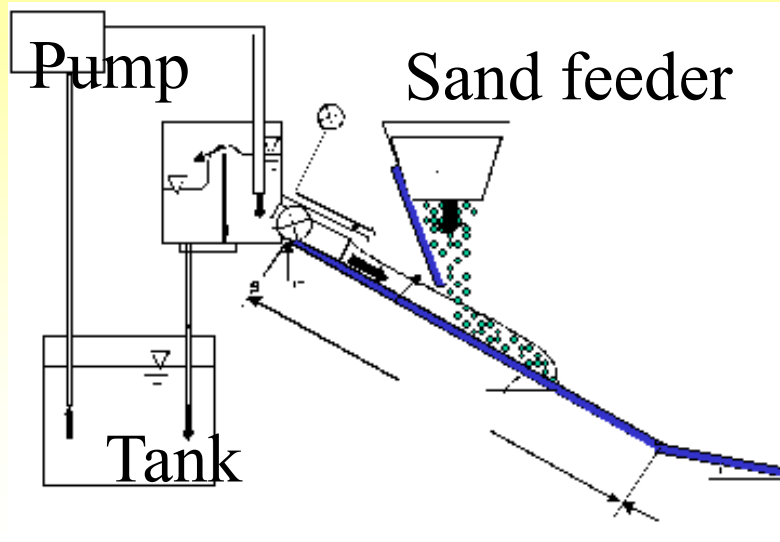
土石実堆積過程に関する実験水路図
