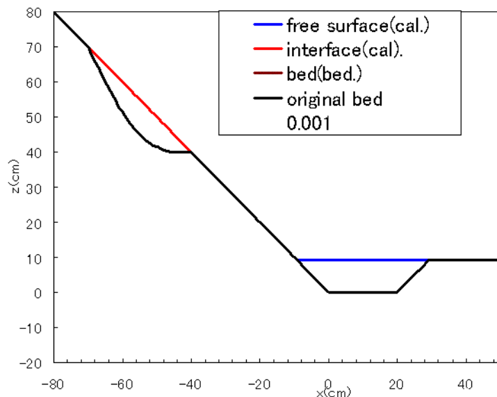
湛水域に流入する土石流
