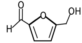
5-ヒドロキシメチルフルフラール
