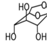
レボグルコサン
